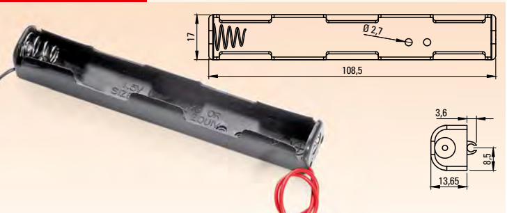
BH-325-1A
